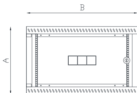
WIDOK ZEW. PRZÓD
